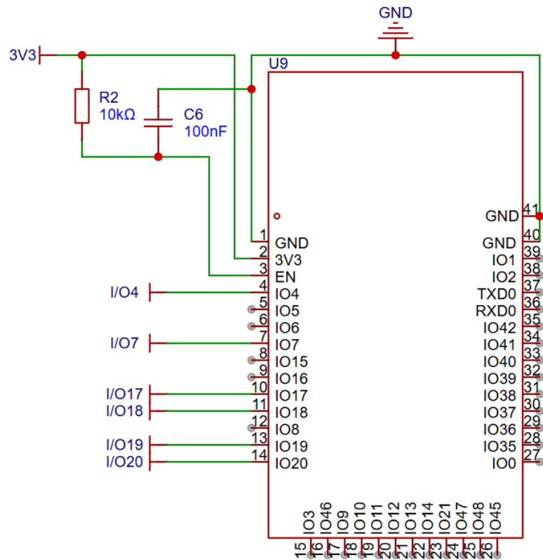
Hình 3.6: Sơ đồ kết nối vi xử lí ESP32-S3
